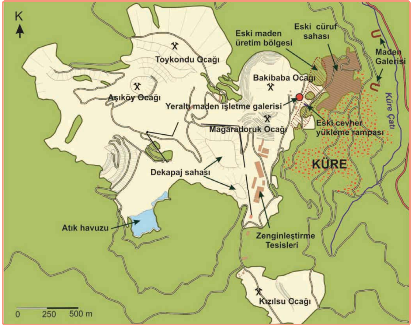
■ Şekil 5. Küre bakır madeni işletme sahasının planı.
